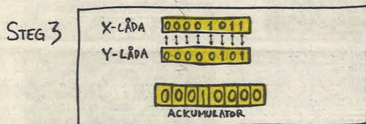
Steg 3: Innehållet i X- och Y-registret jämförs och beräknas binärt. Resultatet läggs i processorns ackumulator-register.
